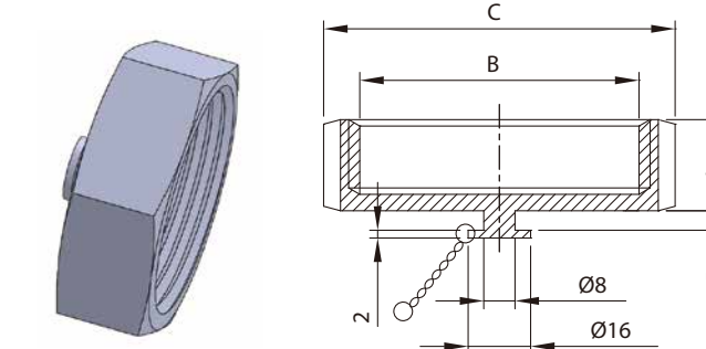
RJT-13HBN Hex.blank nut
