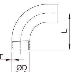
90° Long Elbow
